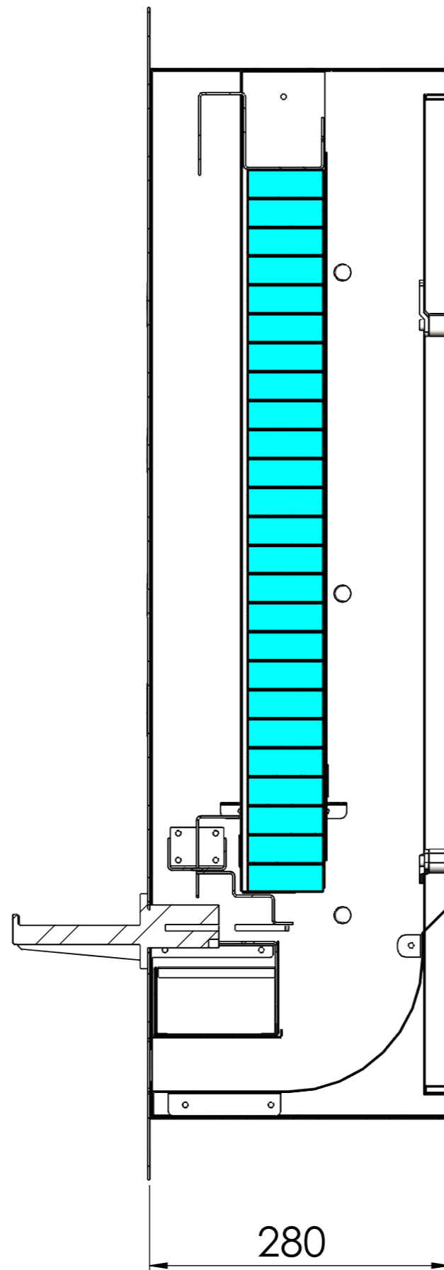
SECTION A-A
